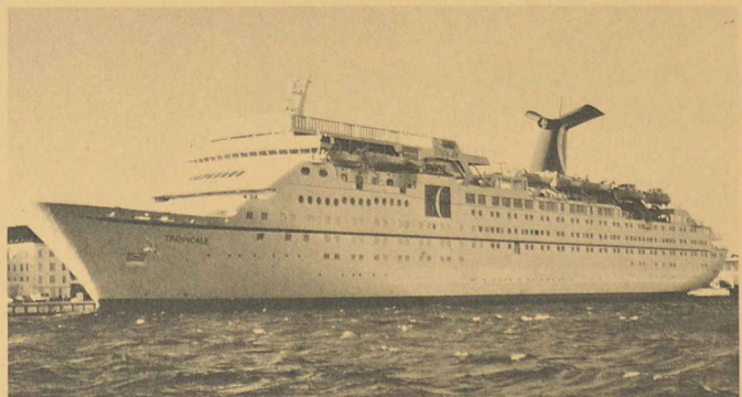
«Tropicale» (30 000 tjb) des Carnival Cruise Lines, équipé de 2 moteurs diesel Sulzer à crosse, à marche lente, développant une puissance totale de 19 560 kW (26 600 ch).
