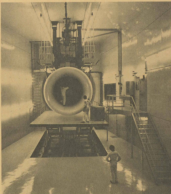
Réacteur à double flux sur son banc d'essais.
