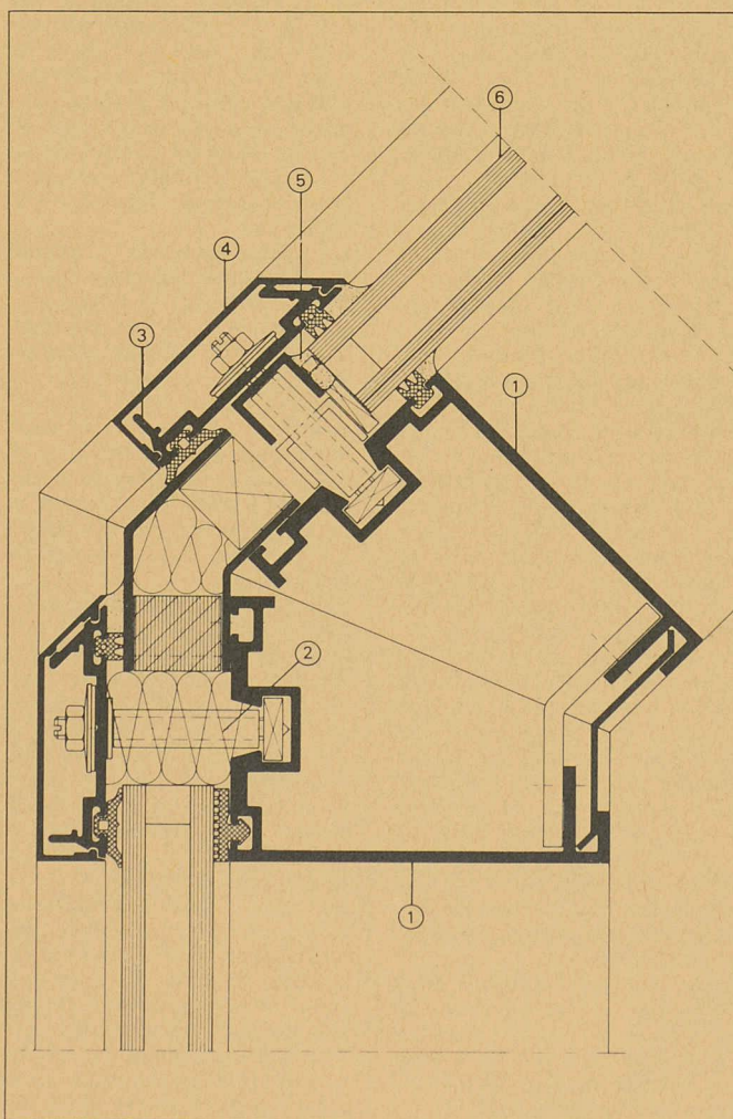
Coupe verticale d'un vitrage oblique AS-200
