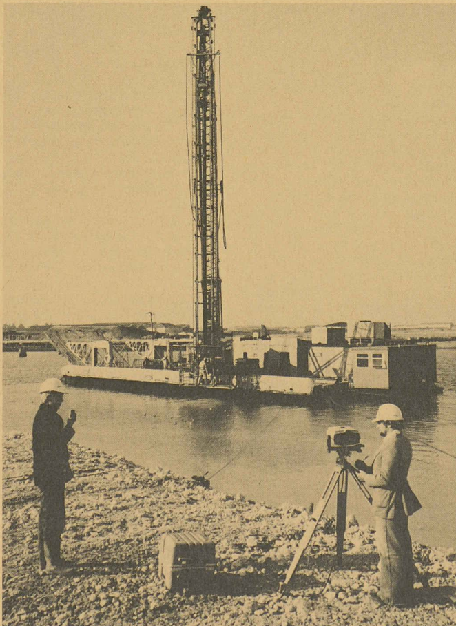
Environ 6000 drains à mèche gainés du géotextile «Tygar» en polypropylène ont été installés sous l'eau par Cementation Ground Engineering au moyen de ce dispositif à mandrin monté sur le ponton. L'emploi du «Mebradrain» diminue la période de consolidation avant de commencer la construction d'un talus pour faire passer de manière économique un pont au-dessus de ce bassin de radoub.
