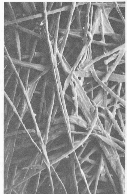
Fig. 3. — Liaison chimique.
