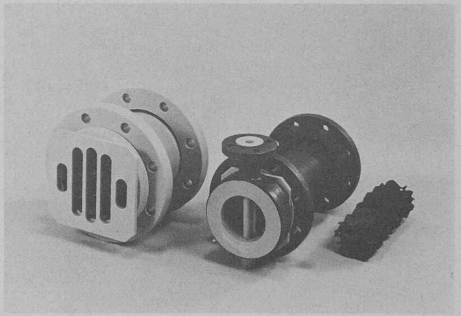
Mélangeurs Sulzer SMV DN 150 en polypropylène (à gauche) et DN 100 avec dispositif d'injection d'additif (à droite). Tube mélangeur et dispositif d'injection d'additif en acier au carbone avec revêtement interne en polypropylène, éléments mélangeurs en polypropylène renforcés par des fibres de verre.
