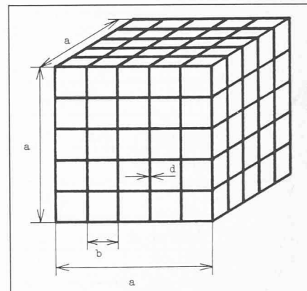
Fig. 9. — Maquette constituée d'armatures. a dimension extérieure de la maquette b distance entre armatures d diamètre d'armatures
