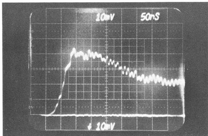
Fig. 6. — Impulsion de champ magnétique mesurée sous l'antenne.
