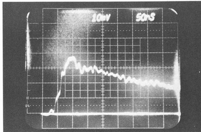
Fig. 8. — Impulsion de champ électrique mesurée sous l'antenne.
