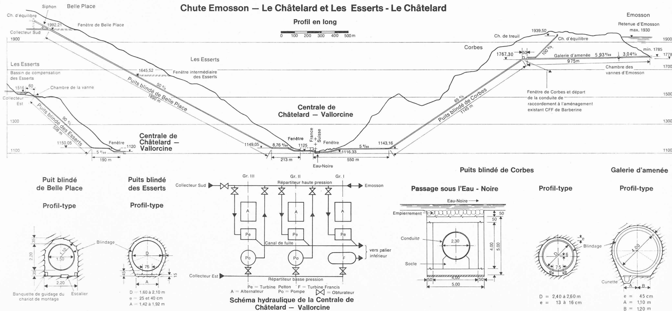
Fig. 13 — Chutes Eמושon-Le Châtelard et Les Esserts-Le Châtelard ainsi que le puits blindé de Belle-Place. Profils en long, profils-types et schéma hydraulique de l'usine de Châtelard-Vallorcine.
