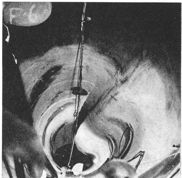
Fig. 9. — Flambage par pression extérieure.
