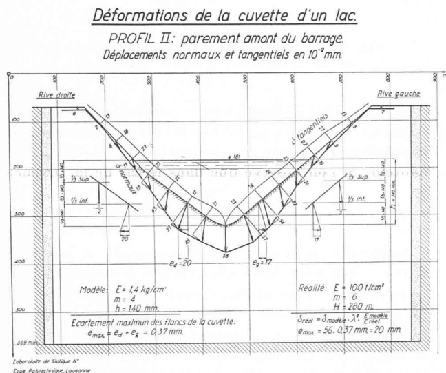
Fig. 21. — Déformation de la cuvette d'un lac le long du parement amont du barrage. Résultat de l'essai.
