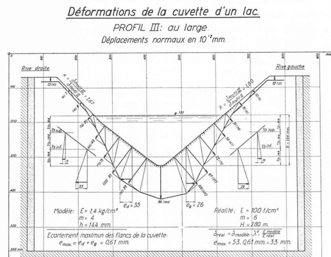
Fig. 22. — Déformation de la cuvette d'un lac à grande distance à l'amont du barrage.
