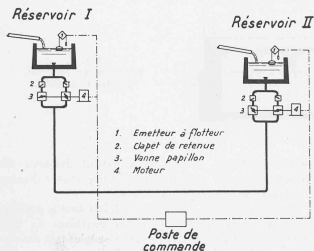
Fig. 6. — Asservissements des installations par commande à distance.
