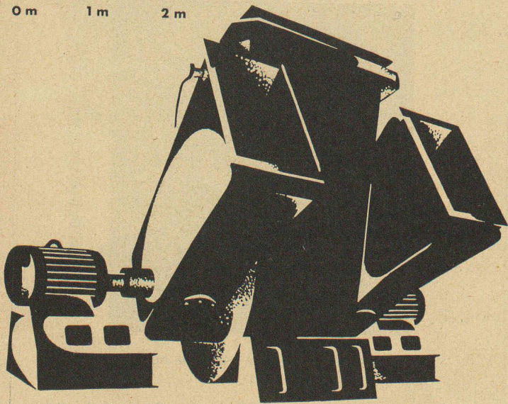
Ventilateur de tirage induit pour une installation de chaudières, Q = 70 m 3 /s ; p = 278 mm eau
