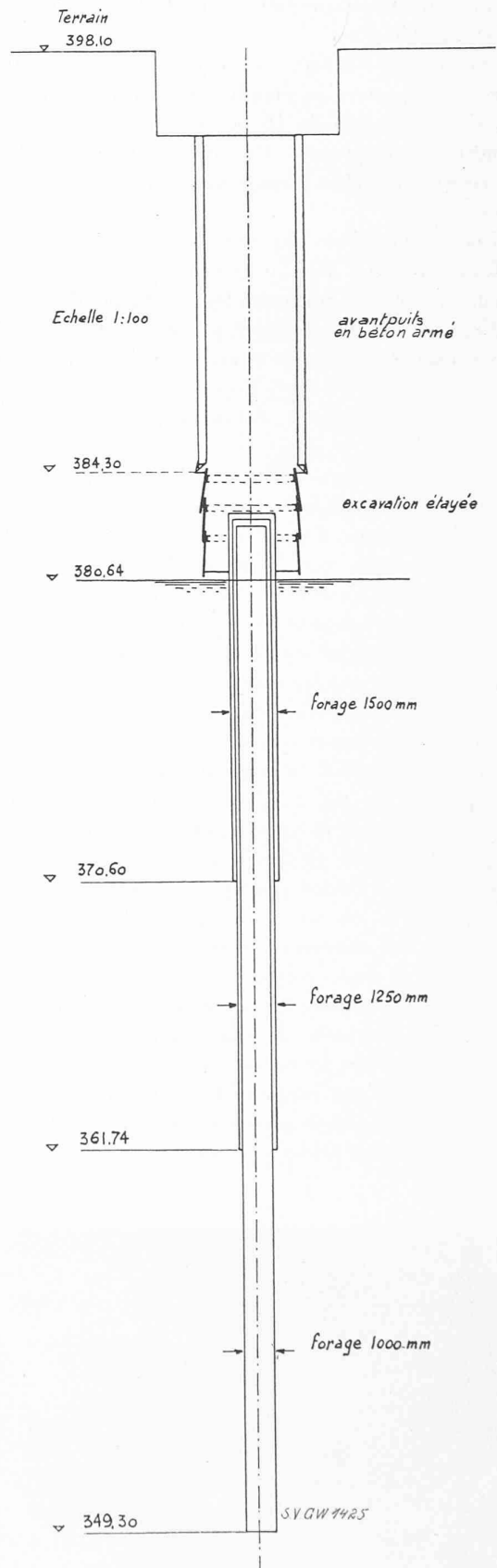
Fig. 5. — Schéma de l'ouvrage en cours d'exécution.
