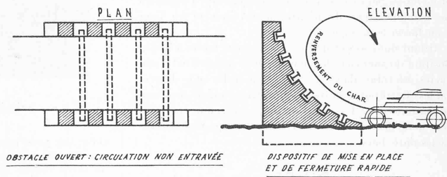
Fig. 7. — Type d'obstacle sur route résistant aux chars de tout tonnage (réaction aux efforts statique et dynamique).
