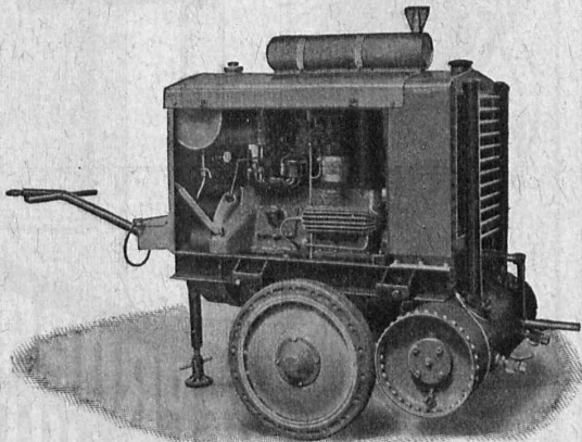
Moteur-compresseur léger type LZ. 20 pour l'actionnement d'un gros marteau perforateur ou d'un brise-béton. Léger, souple, économique.
