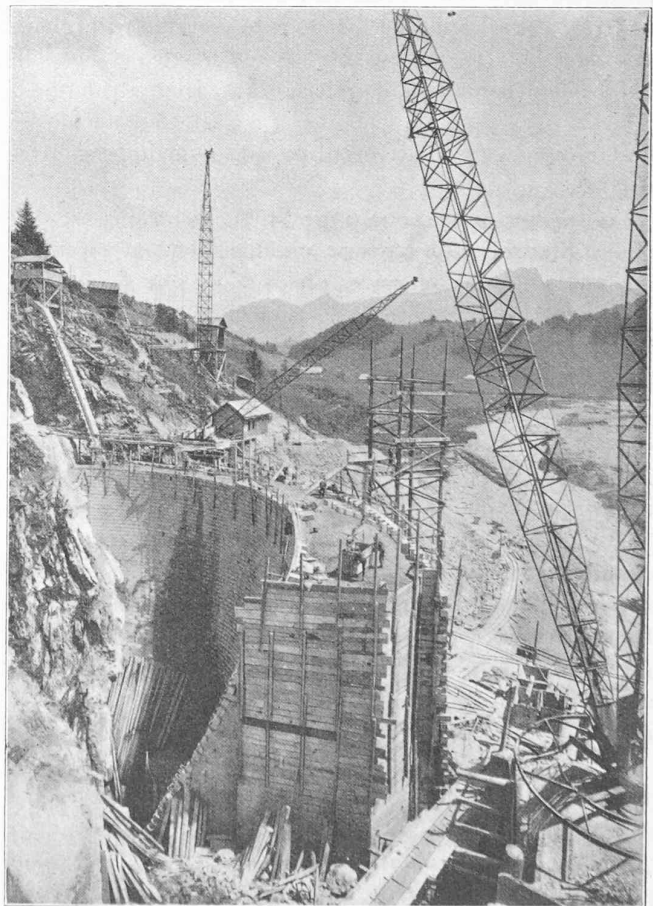
Fig. 12 bis. — Le barrage en construction.
