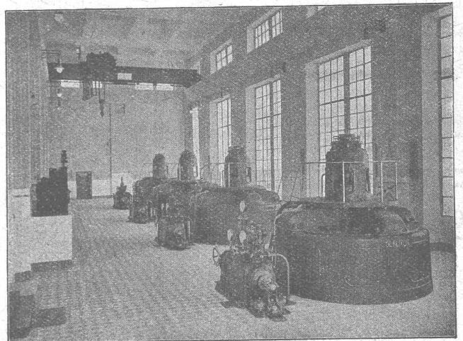
Usine de la Jogne. (Entreprises Electr. Fribourgeoises) 4 turbines de 7800 ch. chacune. Châta: 105-120 m. Vitesse: 500 t/m 1
