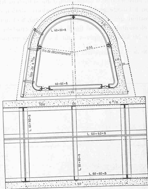
Fig. 17. — Conduite. — 1 : 300.
