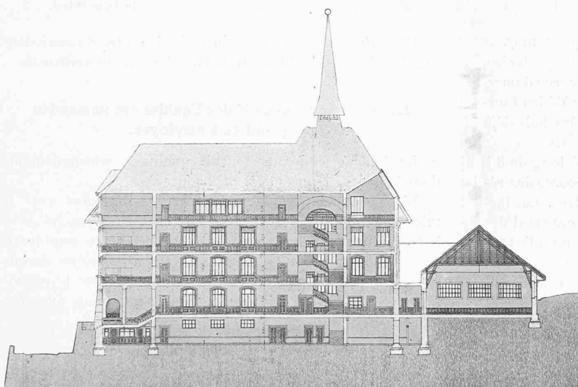
Coupe longitudinale.
