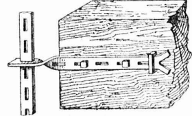
Balkenkopf-Anker
