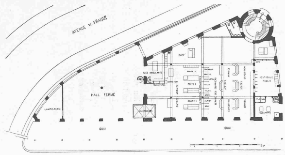
Fig. 2. — Plan du rez-de-chaussée.
