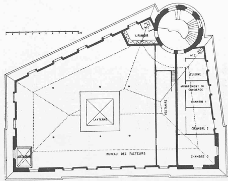
Fig. 4. — Plan du 2 me étage.
