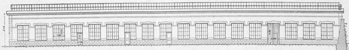
Fig. 24. — Ateliers des Tramways lausannois, en Prélaz. — Façade Nord. — Echelle : 1 : 400.
