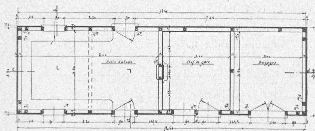
Fig. 18. — Plan d'une gare.
