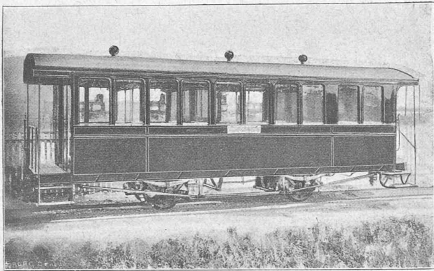
Fig. 25. — Remorque.
