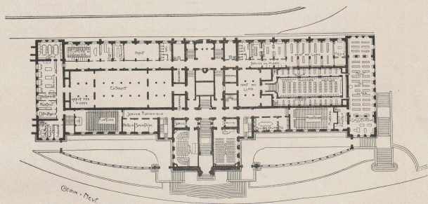
Fig. 5. — Plan du sous-sol.
