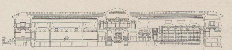
Fig. 8. — Coupe longitudinale. — Echelle : 1 : 600.
