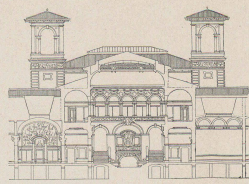
Fig. 9. — Coupe sur l'atrium, Face d'entrée. Echelle : 1 : 600.
