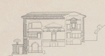
Fig. 10. — Coupe transversale (aile Nord). — Echelle : 1 : 600.
