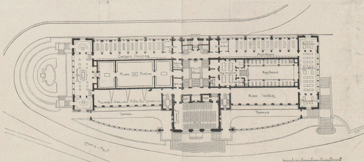
Fig. 6. — Plan du rez-de-chaussée (étage principal).
