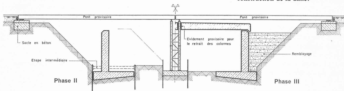
Fig. 185. — Phase II: réalisation des culées. — Phase III: construction de la dalle.
