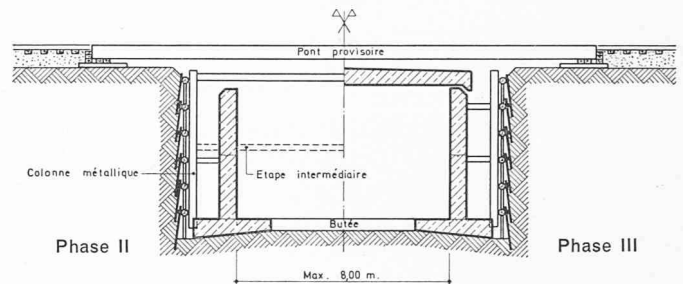
Fig. 181. — Phase II : construction des culées. — Phase III : construction de la dalle.
