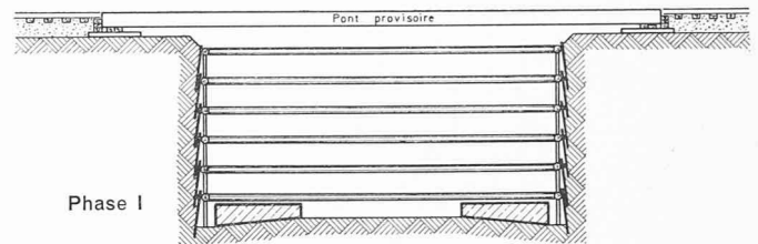
Fig. 180. — Fouille exécutée en marche avant.
