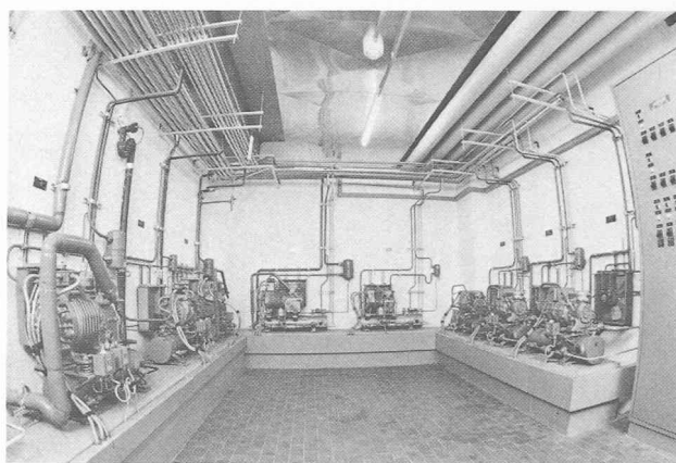
Fig. 15. — Local des compresseurs frigorifiques.
