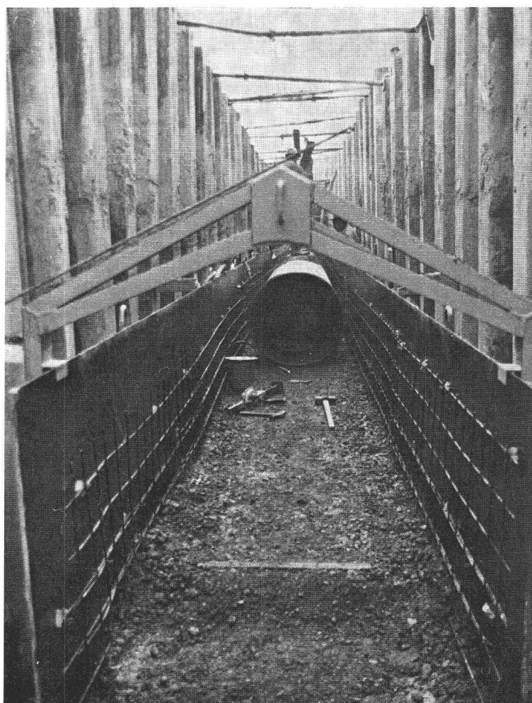
VÉTROZ VS : Emploi d'éléments préfabriqués pour le bétonnage des canalisations en PVC GRESINTEX.
