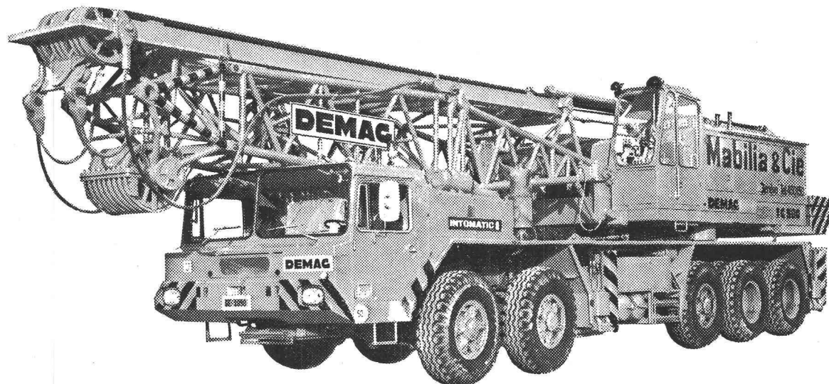
Nouvelle grue DEMAG flèche treillis. Force de levage 140 t. — Hauteur maximum 111 m.
