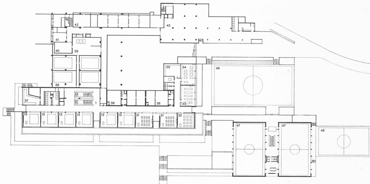
Fig. 8. — Plan du premier niveau inférieur.
