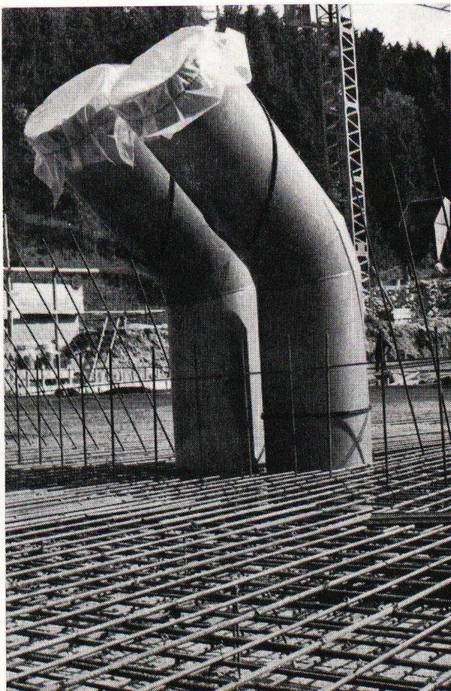
STEP de La Chaux-de-Fonds : Exécution des conduites de liaison avec des tuyaux en PVC GRESINTEX.
