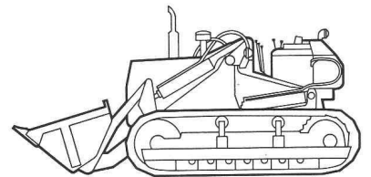
FL 14 Puissance: 140 CV DIN Poids total: 15'400 kg
