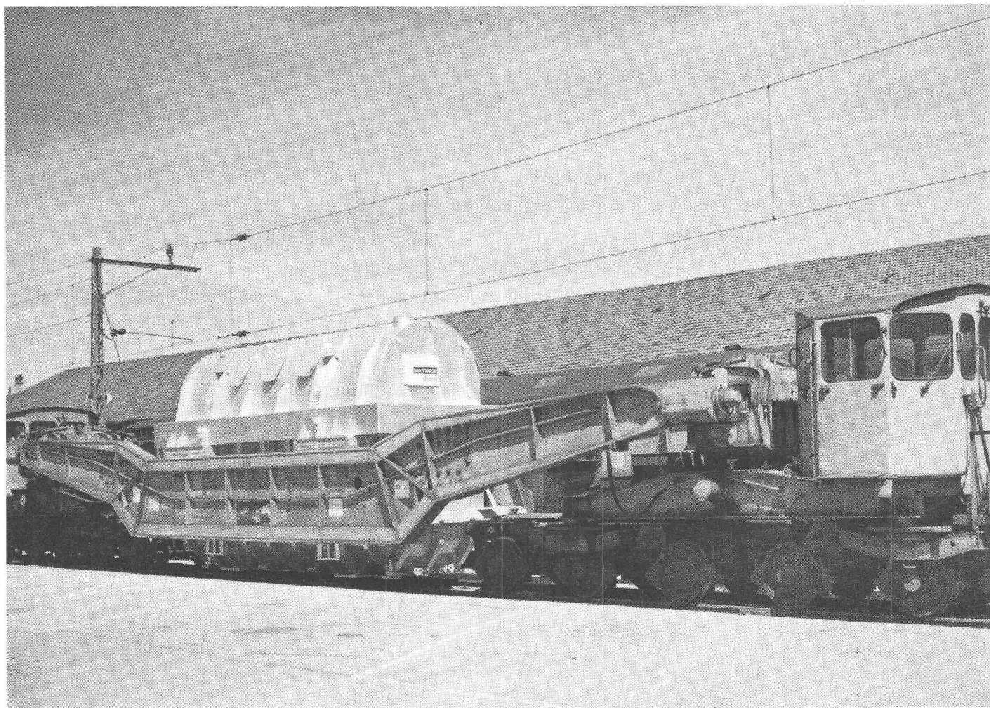
Convoi spécial au départ de Genève avec l'un des deux transformateurs élévateurs triphasés de 220 MVA, 15,5 / 264 \pm 13 kV, 50 Hz, destinés à la Centrale nucléaire de Beznau II, et livrés par les Ateliers de Sécheron à Genève. Le poids de ce transformateur est d'environ de 214 tonnes.
