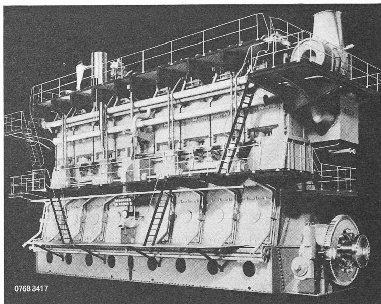
Fig. 1. — Modèle du nouveau moteur Sulzer de 105 cm d'alésage, ayant une puissance par cylindre de 4000 ch. Avec 8 cylindres, le moteur illustré a une puissance totale de 32 000 ch à 108 t/mn.
