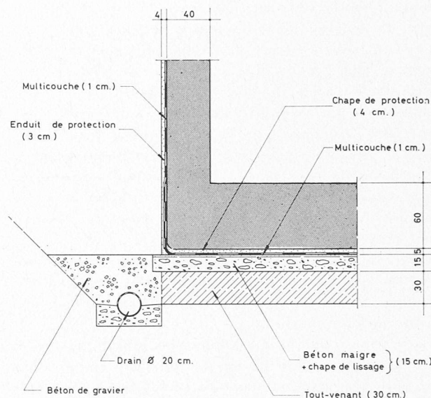
Fig. 2. — Coupe détaillée du sous-radier et du radier.
