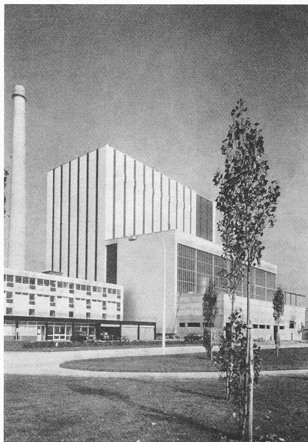
Fig. 2 — Centrale thermique de Blénod-Lès Pont-à-Mousson
