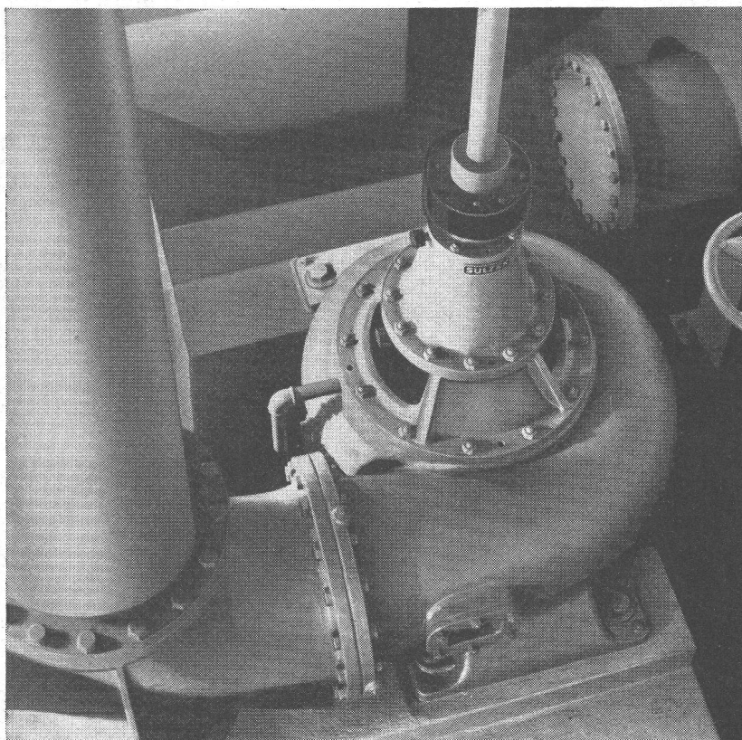
Pompe verticale Sulzer à eaux usées dans la station d'épuration de Küsnacht/Erlenbach. Débit 300 l/s.
