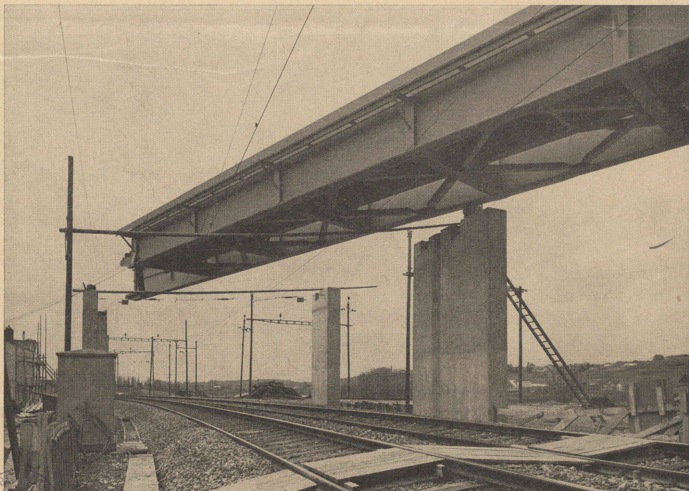
Chemins de Fer fédéraux suisses, 1 er arrondissement. Pont métallique du Saut-de-Mouton du Vertet, entre Renens et Denges (en cours de lancement). Exécution ZWAHLEN & MAYR S. A., Lausanne,
