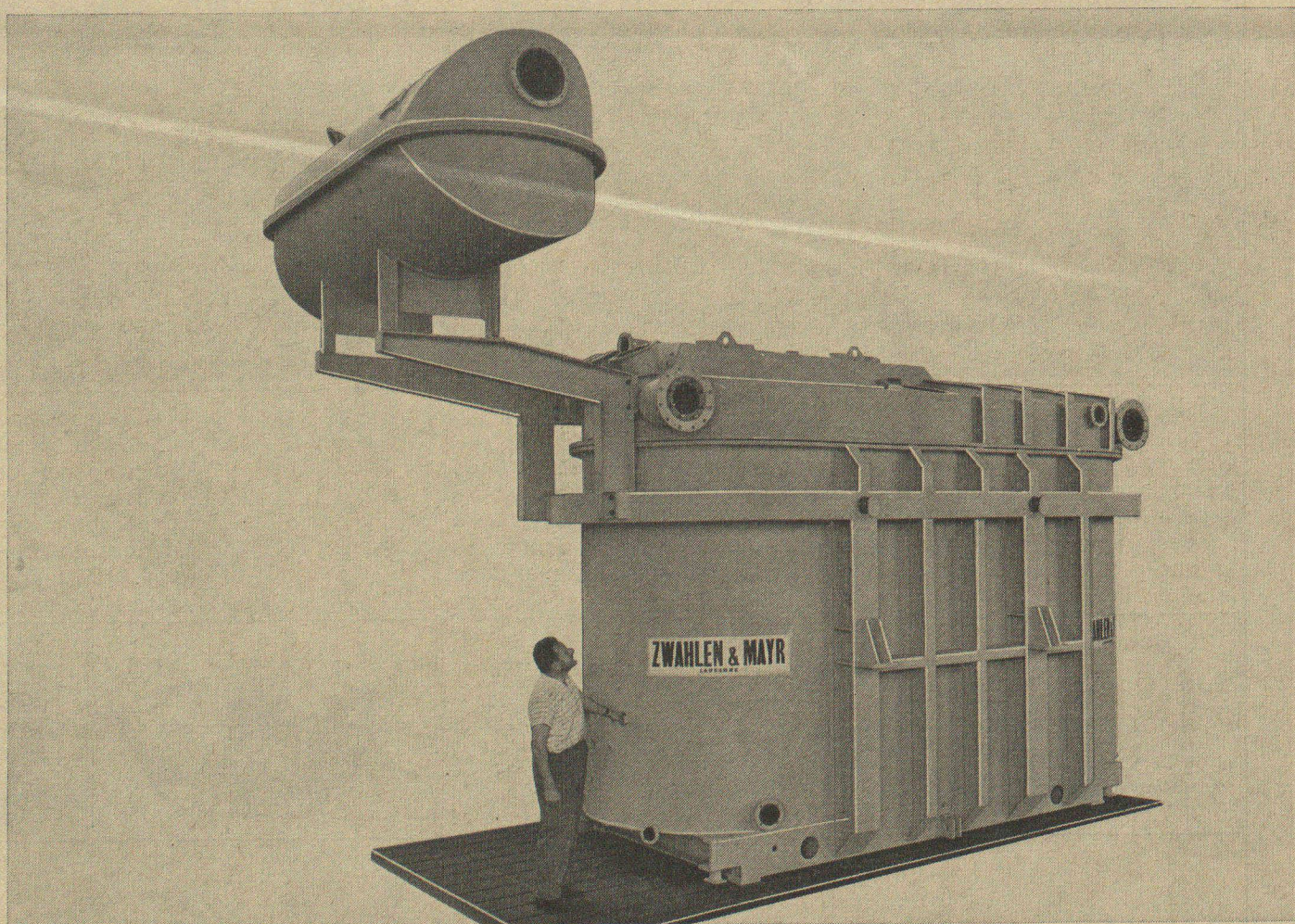
Cuve de transformateur avec conservateur d'huile. (Ateliers ZWAHLEN & MAYR S. A. Lausanne.)
