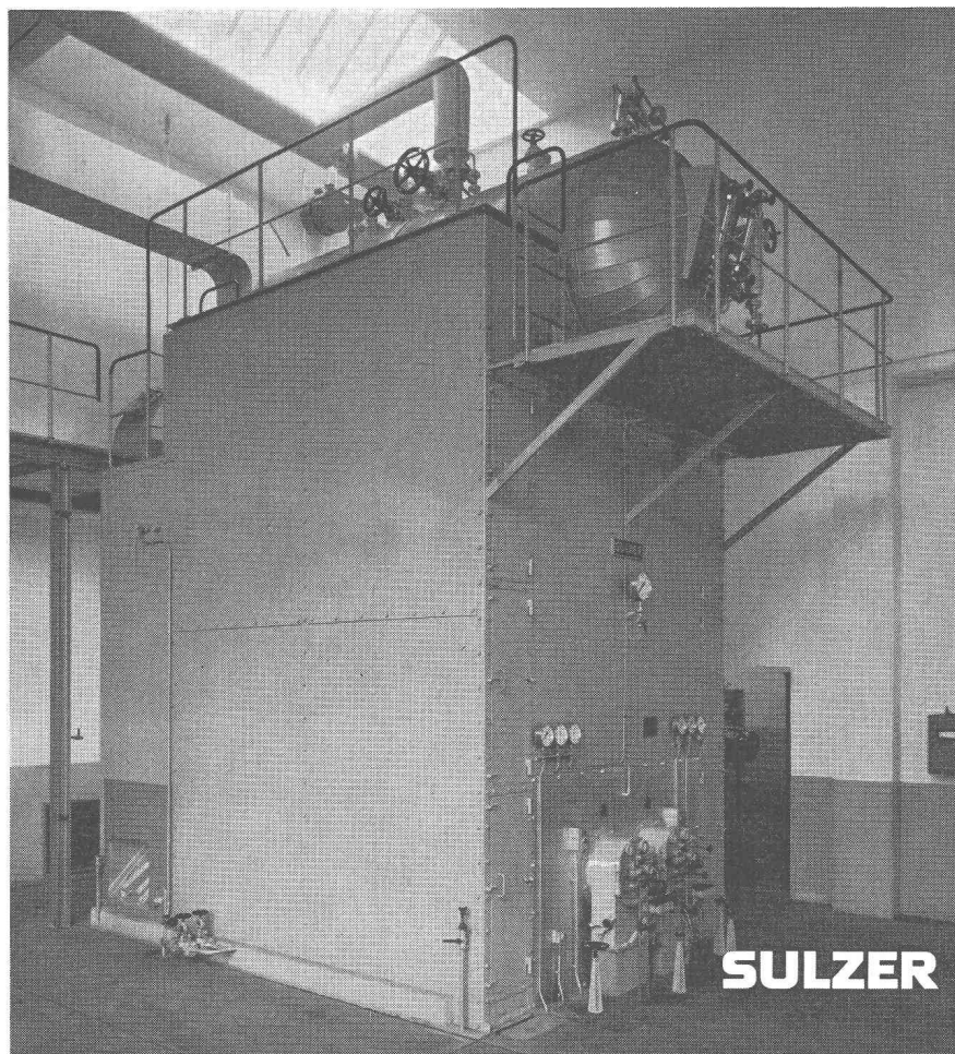
Chaudière à rayonnement Sulzer, type C, de 13 \text{ kg/cm}^2 et 3,2 millions Kcal/h, équipée de 2 brûleurs à mazout, dans un atelier de chemin de fer.
