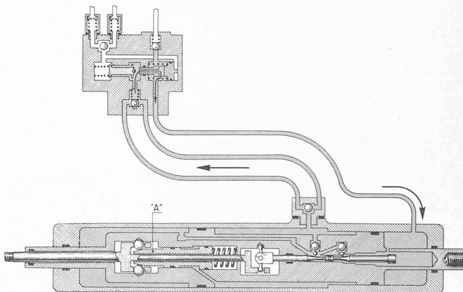
Fig. 2. — Servo-commande « Jacottet-Leduc ». Fonctionnement mécanique.
