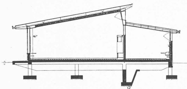
Ecole enfantine — Coupe
