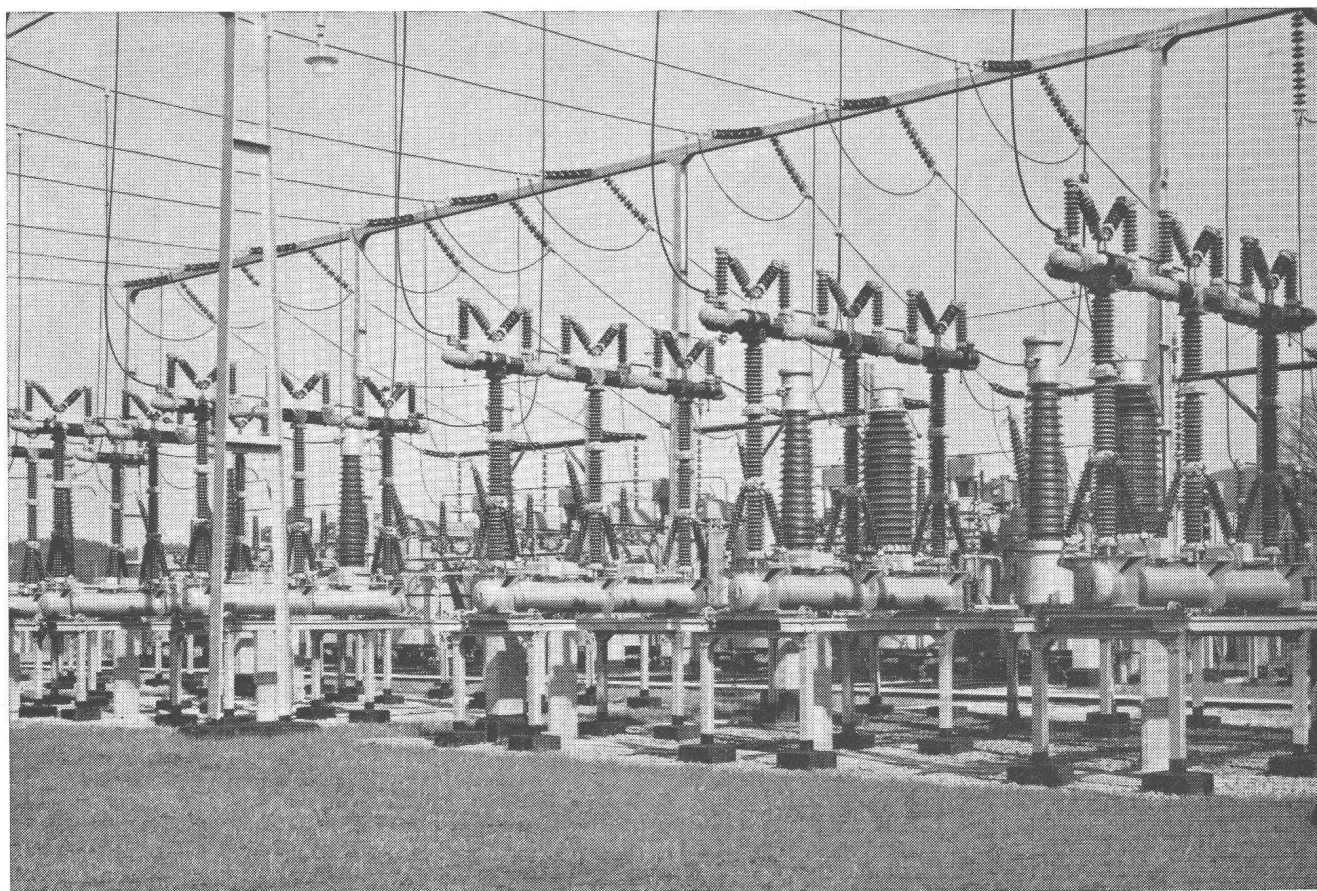
Quatre disjoncteurs pneumatiques ultrarapides Brown Boveri à 220 kV sont en service au poste d'interconnexion de Mettlen, près de Lucerne, où passent les premières lignes du réseau suisse à cette tension.
