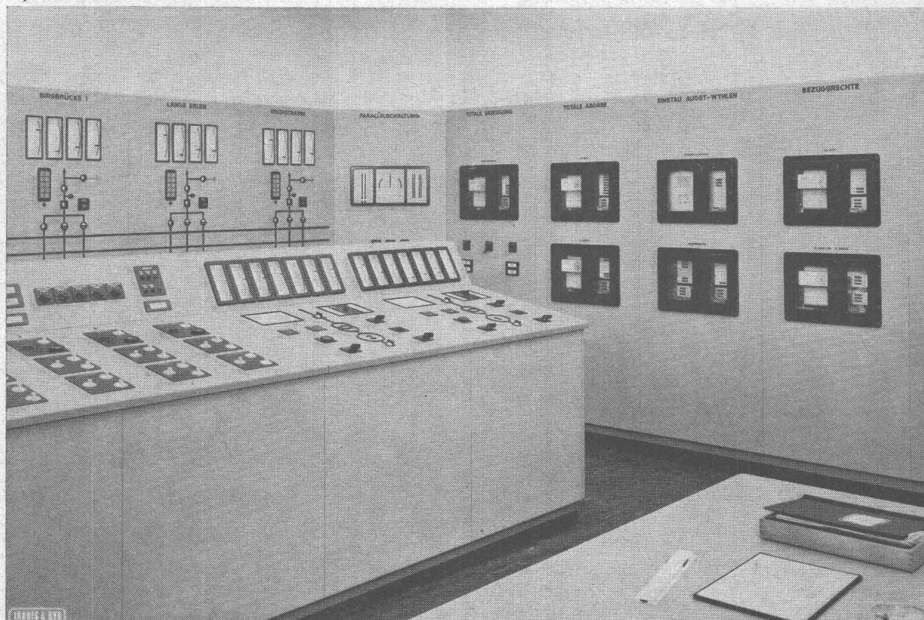
Installation de comptage de l'usine hydroélectrique de Birsfelden (Livraison Landis & Gyr S.A., Zoug).
