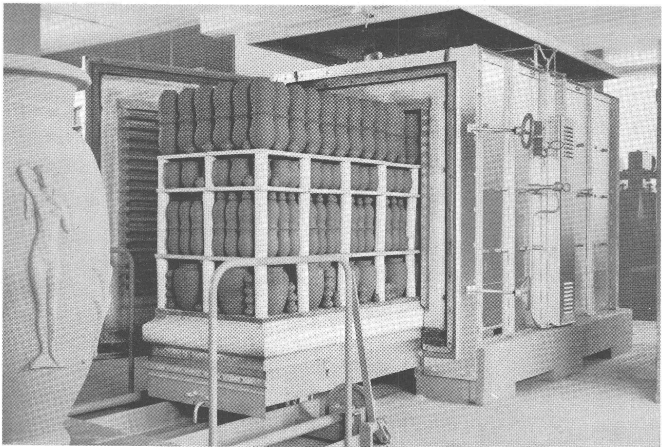
Four électrique Brown Boveri à chariot d'une capacité utile de 2,4 m 3 pour une température maxima de 1300 °C (montre de Seger n° 10)
