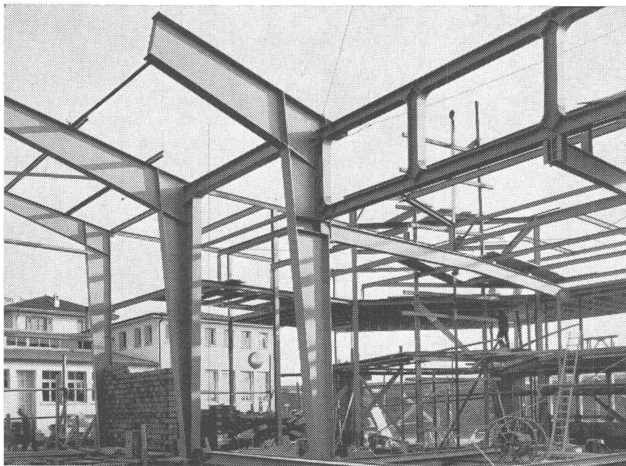
Ossature bâtiment industriel (Garage FBW, Prilly)
