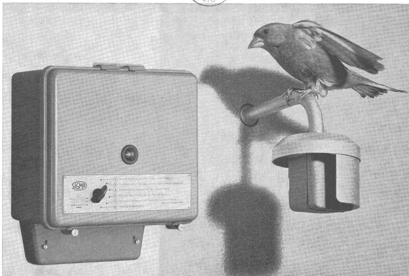
Régulation automatique de chauffages centraux « Sigma » de Landis & Gyr S. A., Zoug. A gauche : le régulateur de pression — A droite : la sonde extérieure (déperditeur)
