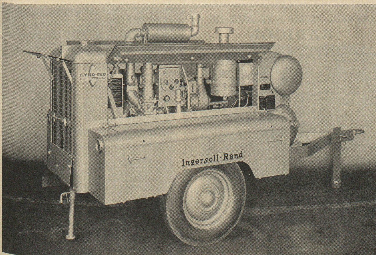
Compresseur transportable INGERSOLL-RAND « Gyro-Flo ». Rendements eff. p/min. 3,6 et 6 m 3
