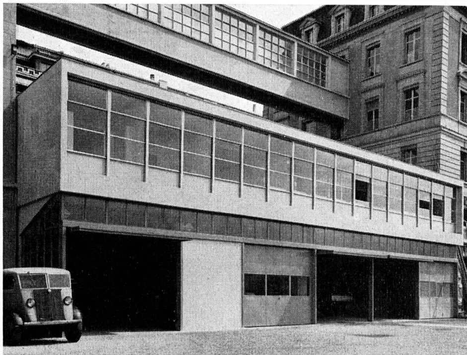
Eléments de vitrages en métal léger pour façades Système à doubles guillottes s'ouvrant simultanément
