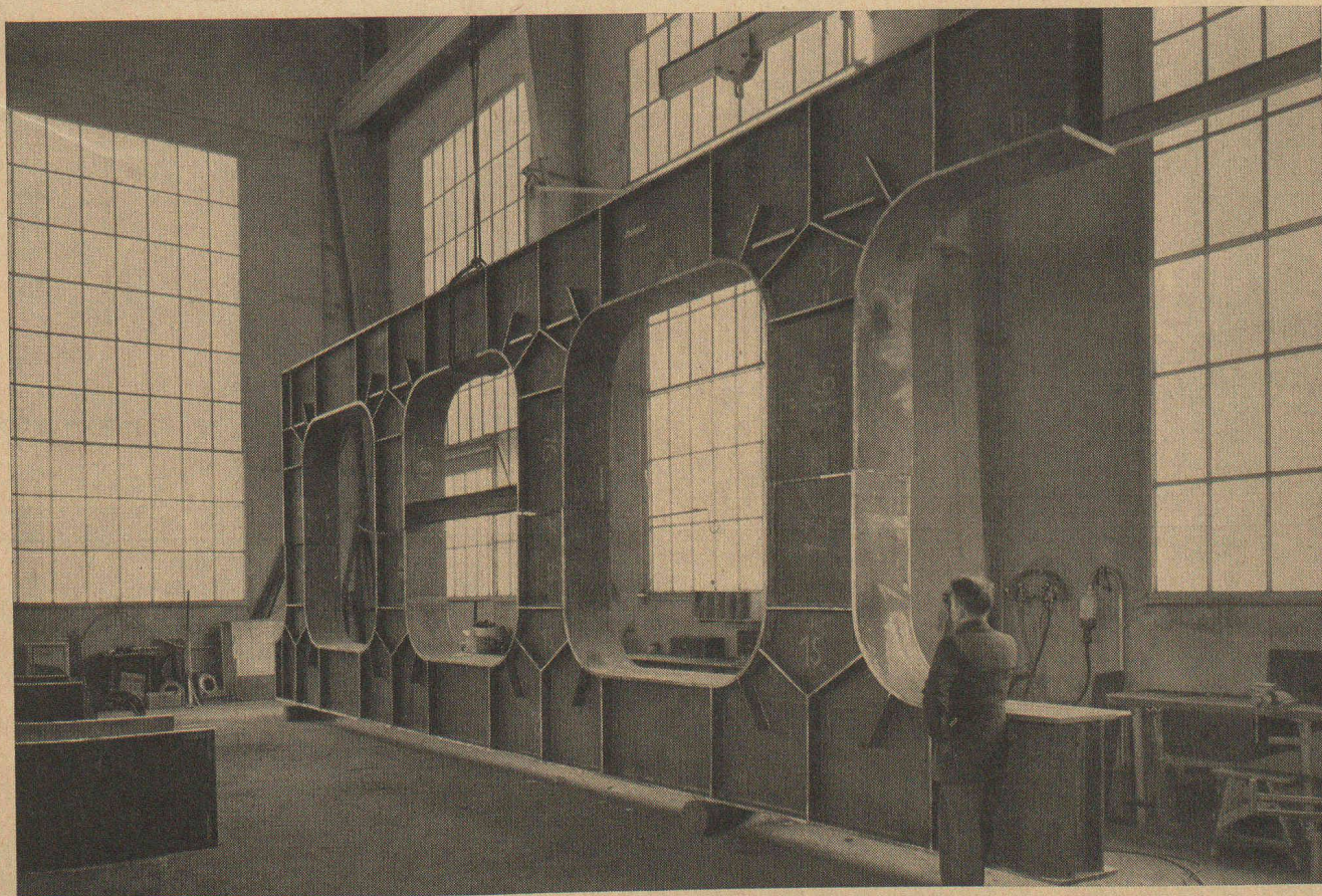
Poutre Vierendeel en acier « LD » exécutée par Zwahlen & Mayr S. A.
