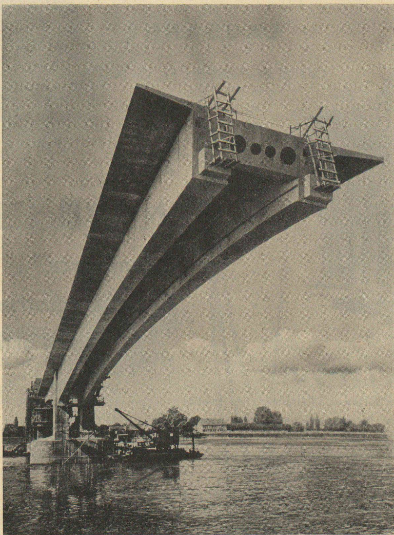
Nibelungenbrücke Worms : Béton précontraint avec adjonctions de PLASTIMENT. Système Dyckerhoff et Widmann.
